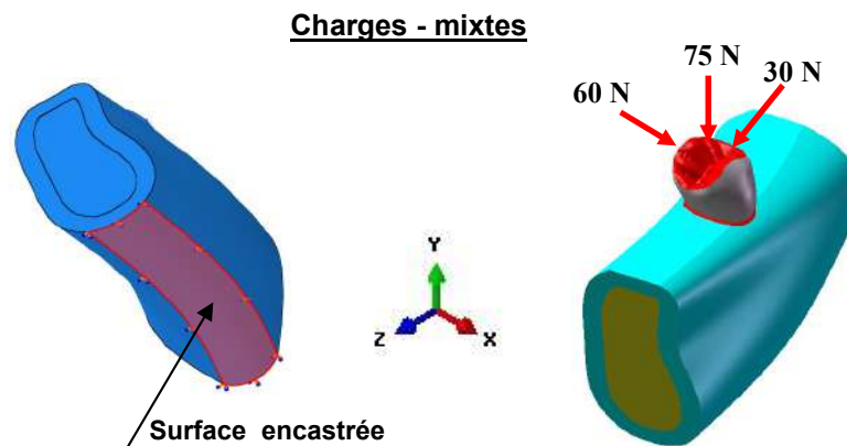
Figure. 4– Conditions aux limites et type de chargement
