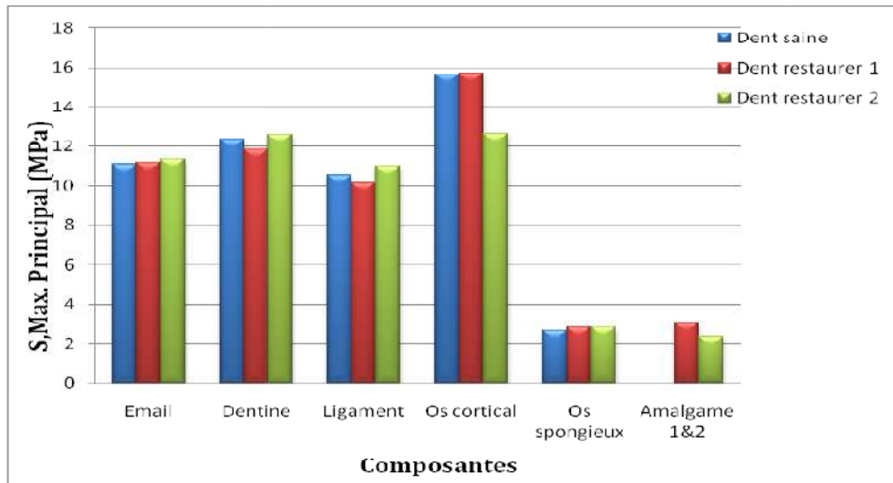
Figure. 13– Histogrammes des contraintes maximales principales pour chaque composant dans les trois modèles sous des chargements mixtes.
