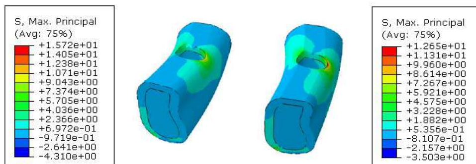
Figure. 11– Distribution des contraintes maximales principales dans l'os pour les deux modèles restaurés.
