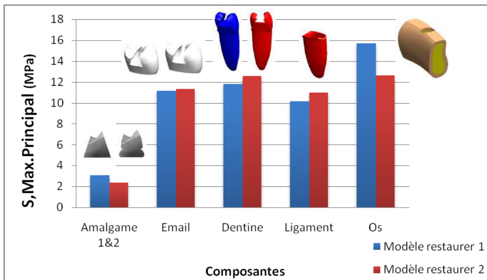
Figure. 12 – Histogrammes des contraintes Max. Principal max pour chaque composante dans les deux modèles sous des chargements mixtes.
