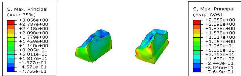
Figure. 7 – Distribution des contraintes Maximales Principales dans l’amalgame pour les deux modèles restaurés.
