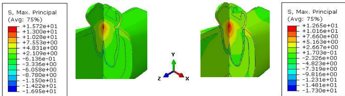
Figure. 6 – Distribution des contraintes principal max dans tous les corps pour les deux modèles restaurés.
