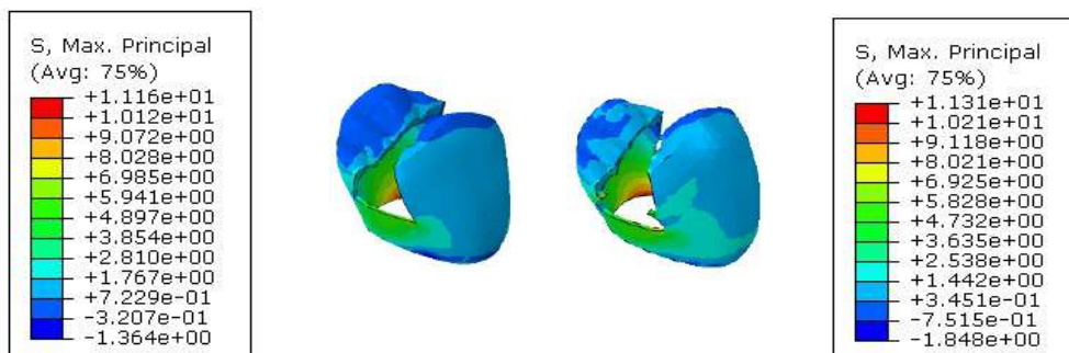
Figure. 8 – Distribution des contraintes Maximales Principales dans l’émail pour les deux modèles restaurés.
