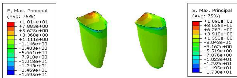
Figure. 10 – Distribution des contraintes maximales principales dans le ligament pour les deux modèles restaurés.
