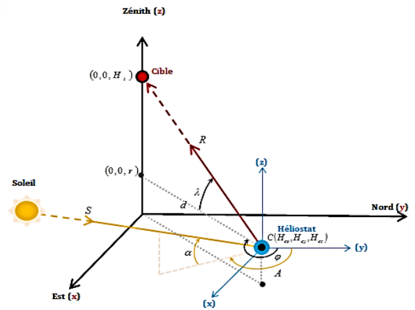
Fig.2 Rayons incident et réfléchi [6].
