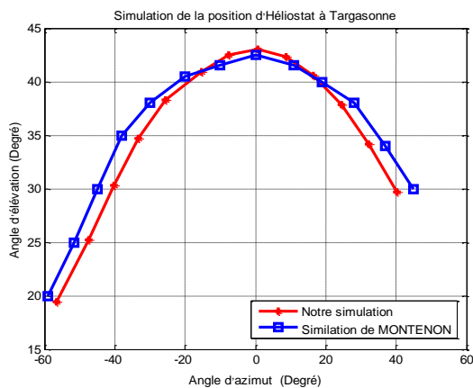
Fig. 4 Validation de notre modèle de poursuite de la méthode (AE) avec ceux utilisé par MONTENON [16] à 21 Juin pour Targastonne ( \theta = 42.45^\circ , L=1.44^\circ ), \lambda = 15^\circ , \varphi = 0^\circ
