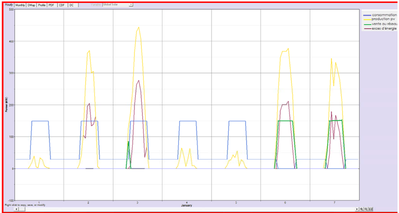
Figure 08- Les résultats de simulation (cas global)
