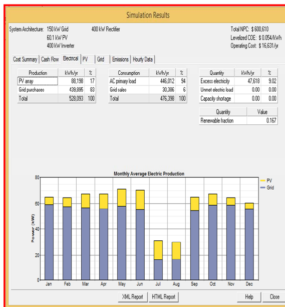
Figure 06- Les résultats de simulation (cas 01)
