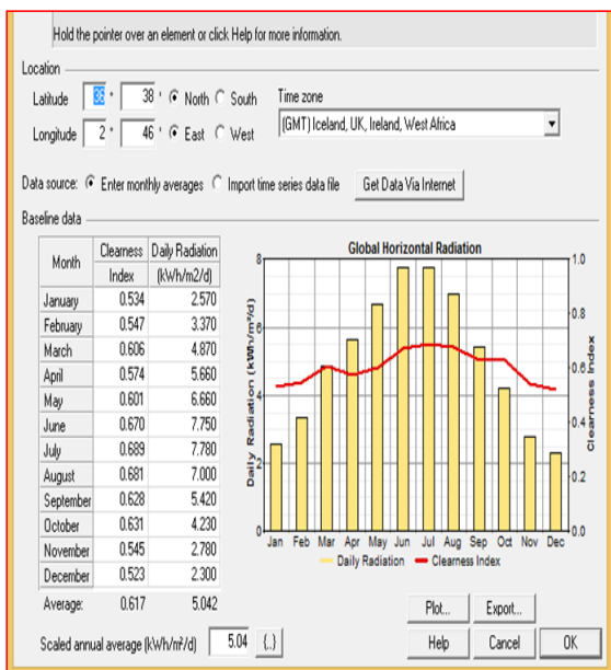
Figure 05- Les données des ressources solaires
