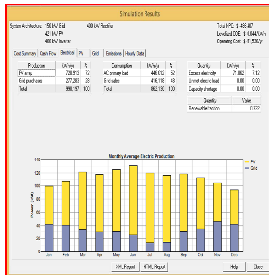
Figure 09- Les résultats de simulation 'cas global)
