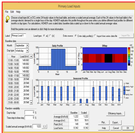
Figure 02- Les détails de charge
