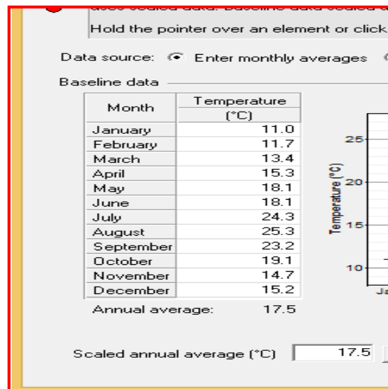
Figure 04- Les températures
