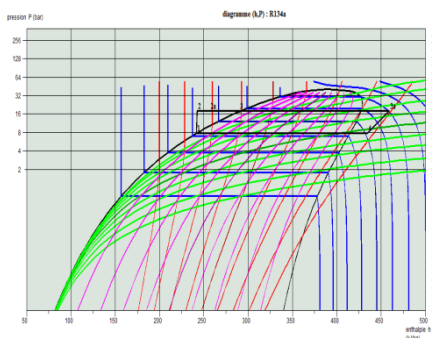
FIG 10. diagramme enthalpie (P.H)
