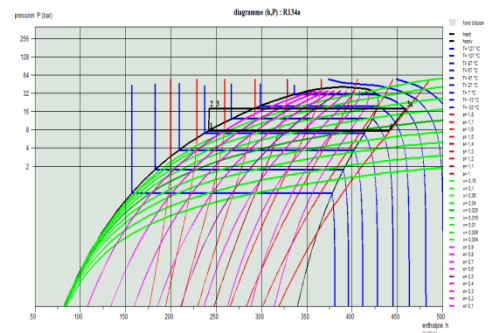
FIG 6. diagramme enthalpie (P.H)
