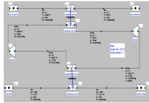
FIG 3. Schéma d'une centrale géothermale simple avec son bilan global
