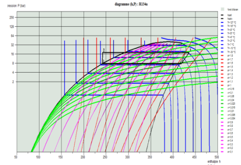
FIG 4. diagramme enthalpie (P.H)
