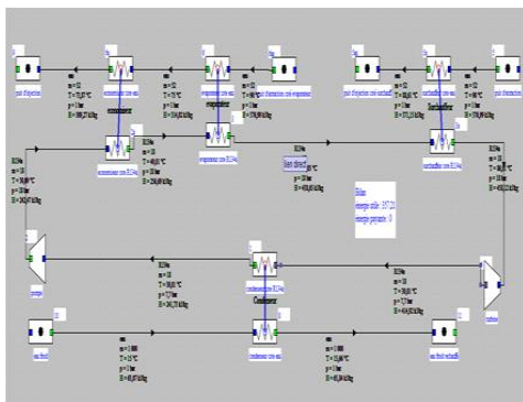
FIG 9 Schéma d'une centrale géothermale avec son bilan global (cycle simple avec économiseur et surchauffeur)
