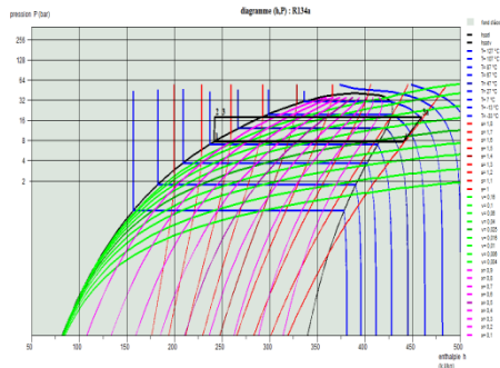
FIG 8. diagramme enthalpie (P.H)
