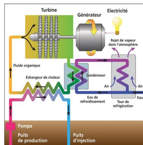
Fig2. Le principe de fonctionnement d'une centrale à vapeur
