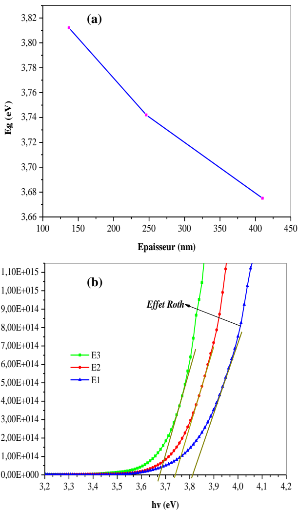
Fig. 3 a) Evaluation du gap optique en fonction de l'épaisseur, b) Shift du gap optique des couches minces de TiO 2 pour différentes épaisseur
